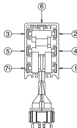
Схема расположения щеток в CL7
