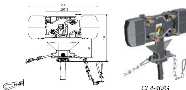
CL4-40/G
