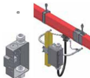
BMV35 + TTB35-4
